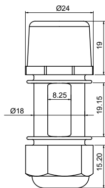
Габаритні розміри датчика до SOU-1/ SOU-2
