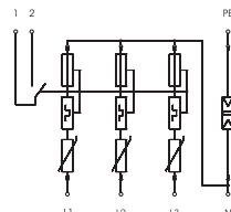
V20-C3+NPE400+FS
