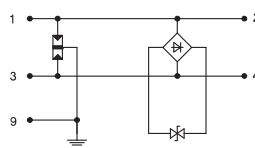
MDP-2 D-24-T-10
