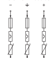
VG-C DCPH1000-6S
