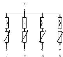
V25-B+C 4-385
