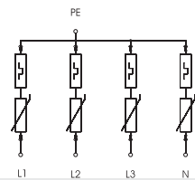
V25-B+C 4-280
