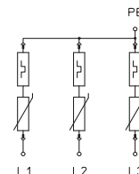
V25-B+C 3-385
